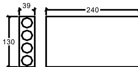
PERFIL ALZADO
